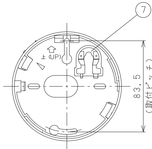
取付寸法図
