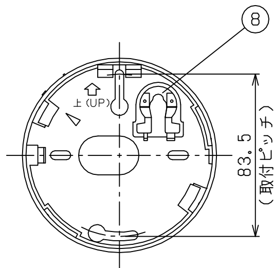
取付寸法図
