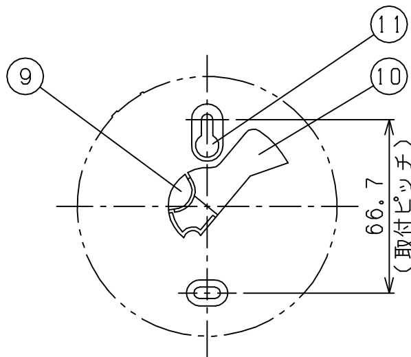
取付寸法図
