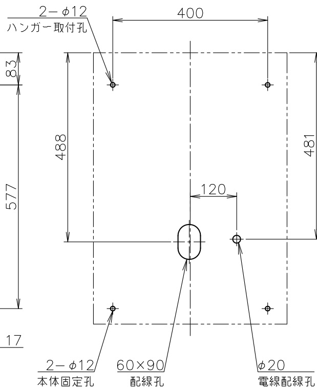
取付寸法図：正面視
